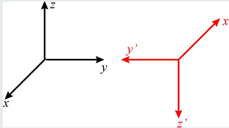
Rysunek 10.1: Inwersja układu współrzędnych w przestrzeni 3-wymiarowej.
